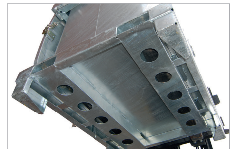
Doorlopende inrijdkokers
