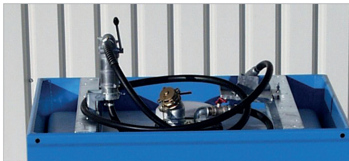
M 800 avec pompe manuelle
