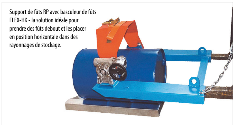
Dépose sur support de fûts RP
