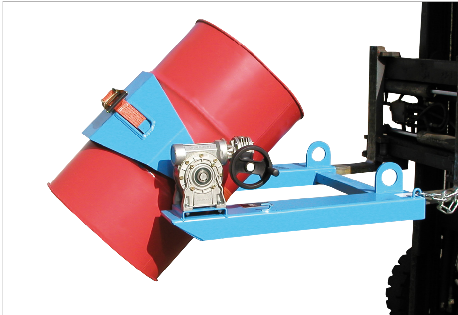
FLEX-HK, déversement d'un fût métallique à bonde de 200 litres
