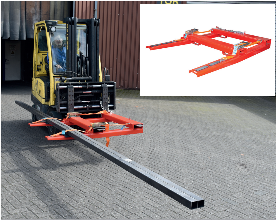
Opnamepositie voor transport b.v. door poorten en gangen
