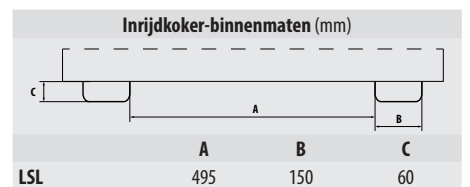
Eenvoudig passeren door poorten en gangen bij het transport van langgoedmateriaal met de LSL
