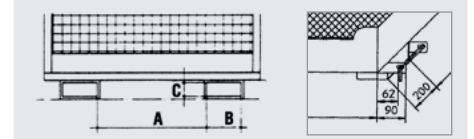
Points d'ancrage pour PSA (EPI)
