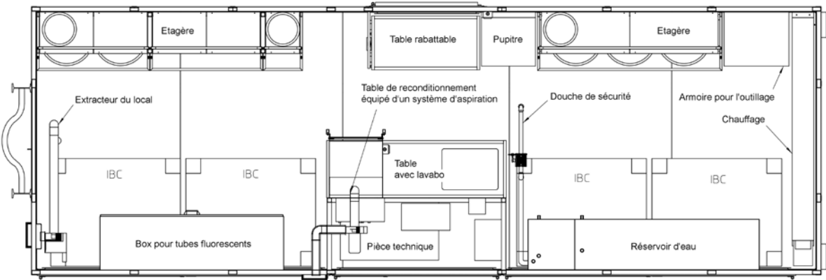
Exemple de structure de base d'un point de collecte mobile
