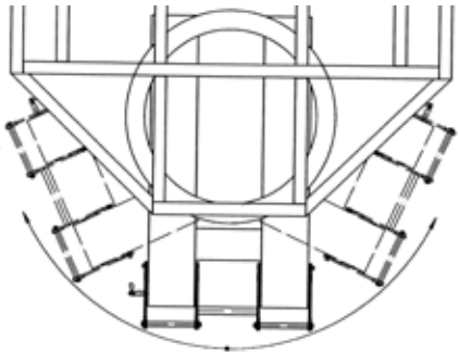
Couronne pivotante à entrées de fourches
