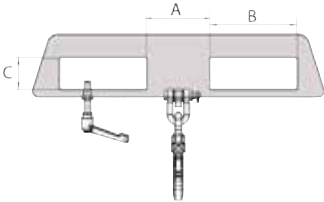
Dimensions intérieures des fourreaux (croquis type LH-II)
