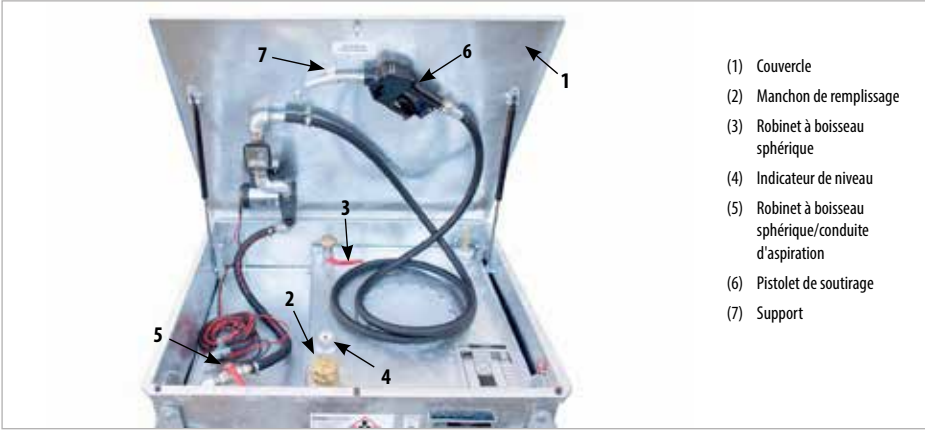
MT 1000 équipé d'une pompe électrique
