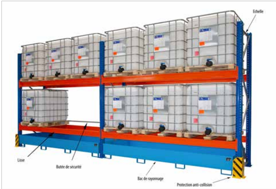
Rack type UR-G 3300 et rack complémentaire type UR-A 3300 avec 2x RW 3300-3, protections anti-collision (en option)
