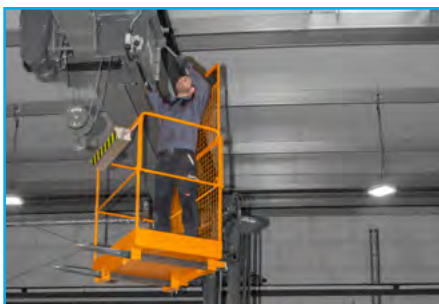
Werkkooien 46-51
