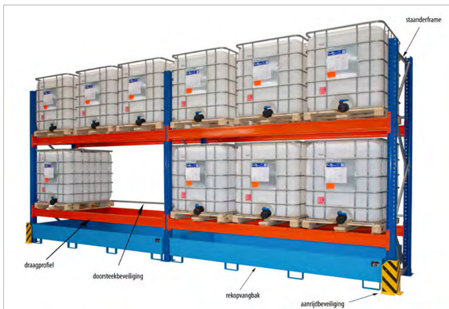
Basisrek UR-G 3300 en aanbouwrek UR-A 3300 met 2x RW 3300-3, aanrijdbeveiliging (optie)
