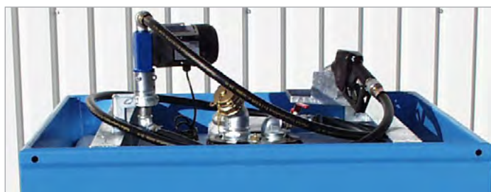
M 800 met elektropomp
