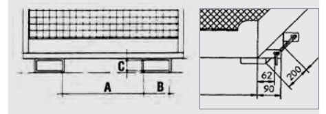
Inrijdkoker-binnenmaten (mm)
